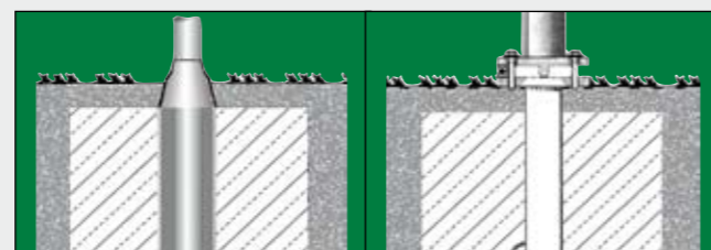
Detailzeichnung: Bodenhülse
